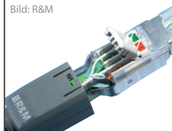
Feldkonfektionierbarer Stecker Connecteur confectionnable sur site
