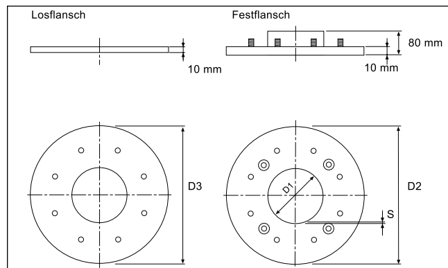
Bemaßung
